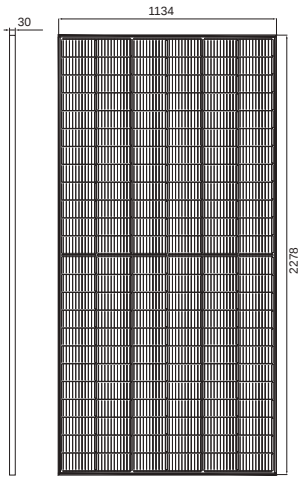
组件正面
