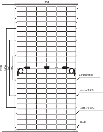
组件背面
